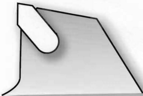
Z型 斜め埋込
